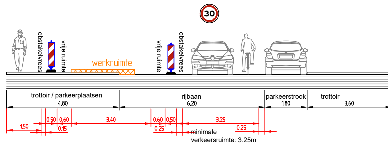
Dwarsdoorsnede A - A
