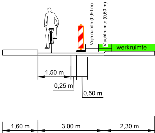
DOORSNEDE A SCHAAL 1:100
