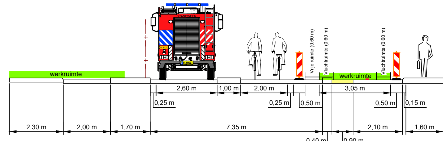
DOORSNEDEN A SCHAAL 1:100
