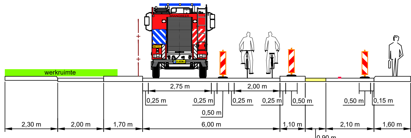
DOORSNEDEN B SCHAAL 1:100
