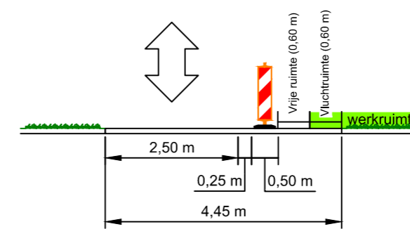
DOORSNEDE SCHAAL 1:100
