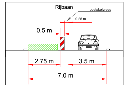
Dwarsdoorsnede A-A
