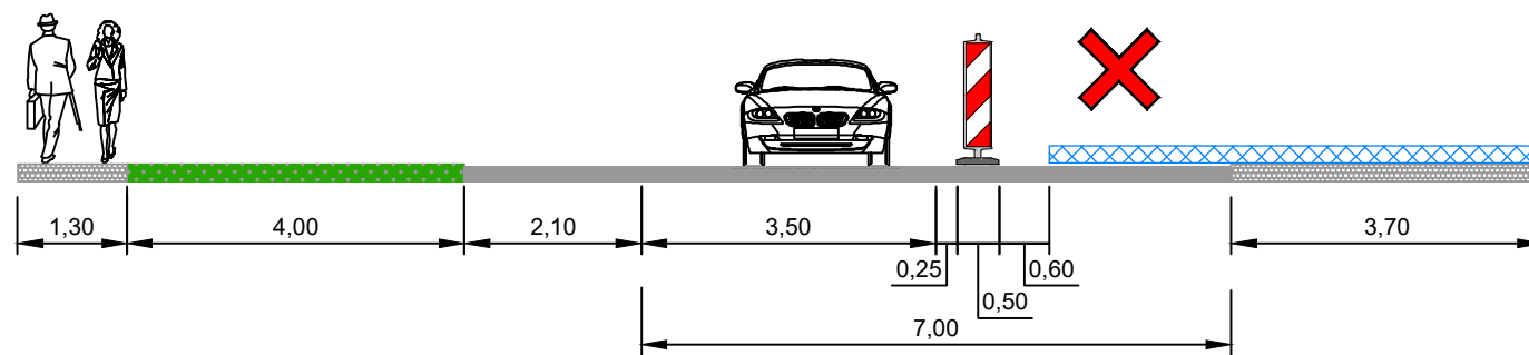
dwarsprofiel B-B
