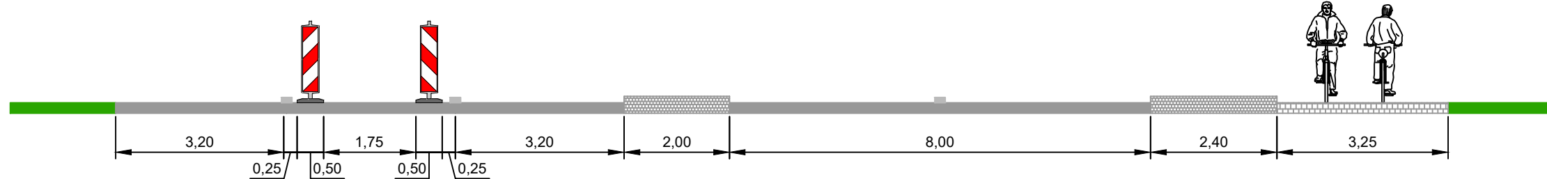
Dwarsprofiel A
