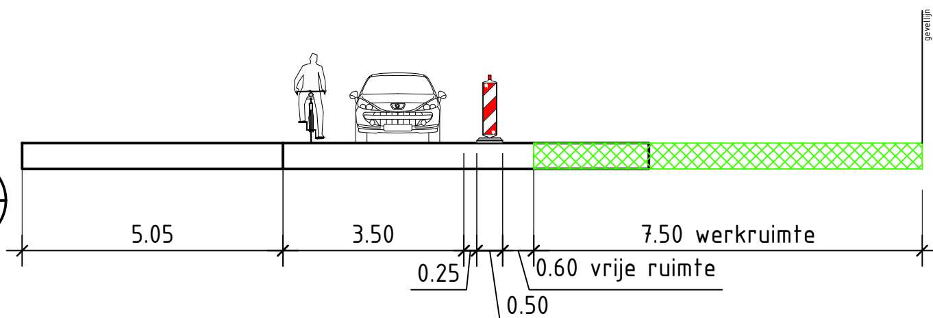
DOORSNEDE A SCHAAL 1:100
