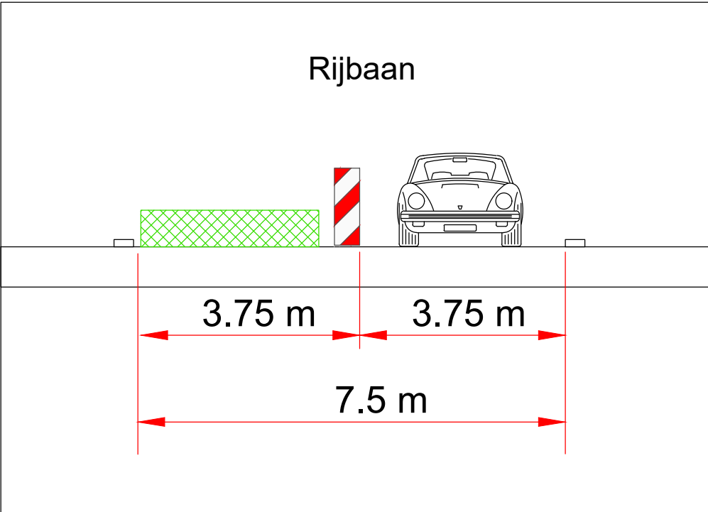
Dwarsdoorsnede A-A
