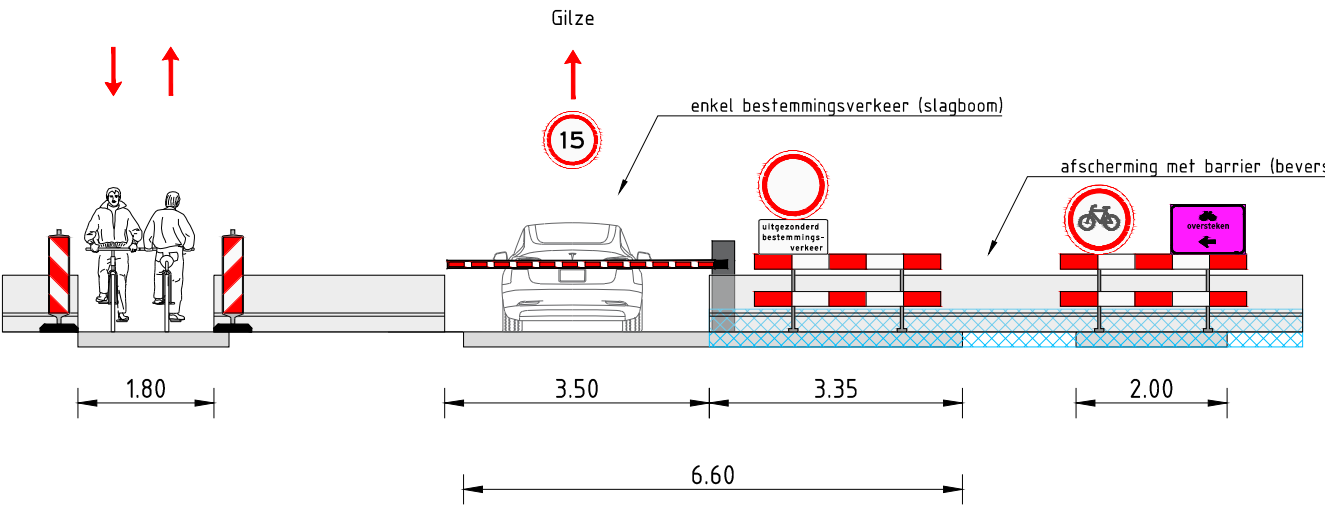
DOORSNEDEN SCHAAAL 1:100
