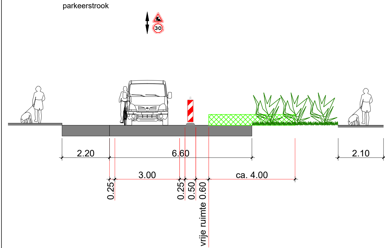
DOORSNEDE A
