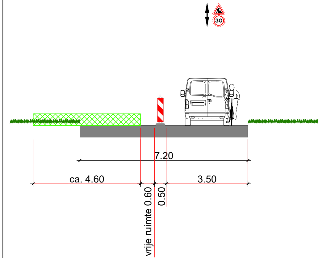
DOORSNEDE A
