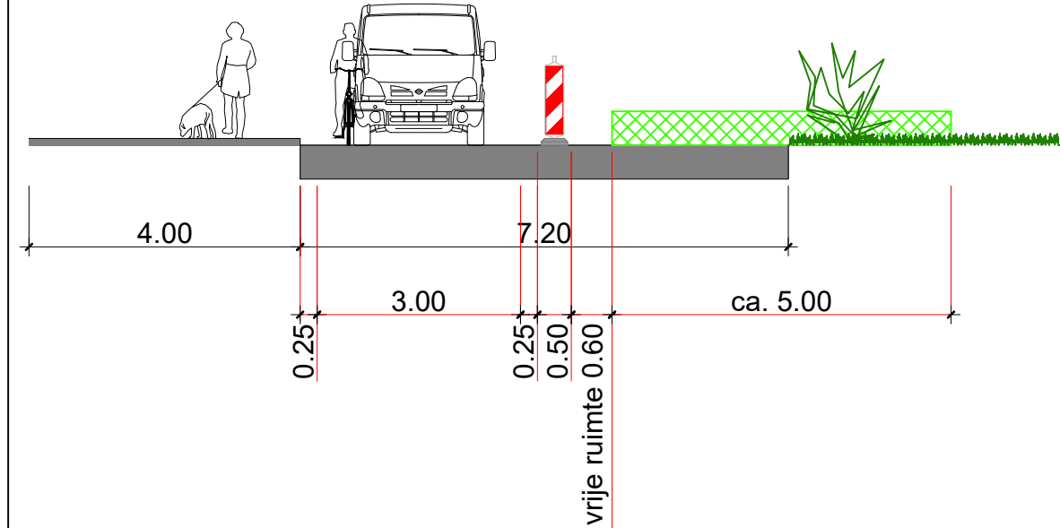
DOORSNEDE A
