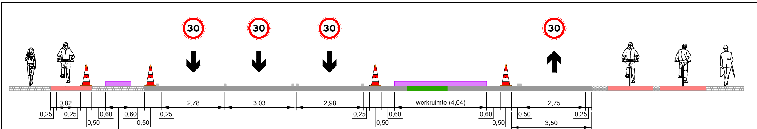
Dwarsprofiel 1 Schaal 1:100
