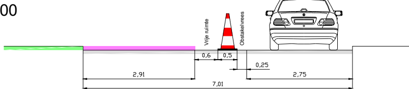
Dwarsprofiel A Schaal: 1:100
