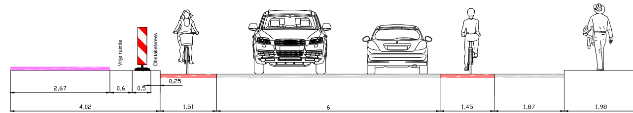
Dwarsprofiel B Schaal: 1:100
