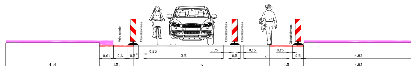
Dwarsprofiel A Schaal: 1:100
