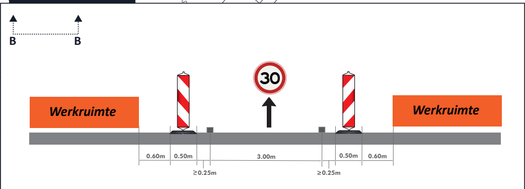
Dwarsdoorsnede B & D
