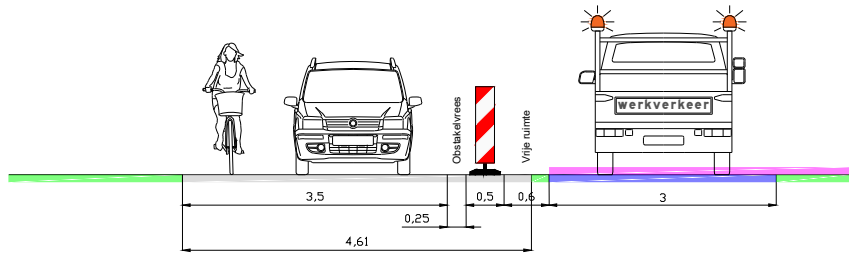
Dwarsprofiel A Schaal: 1:100
