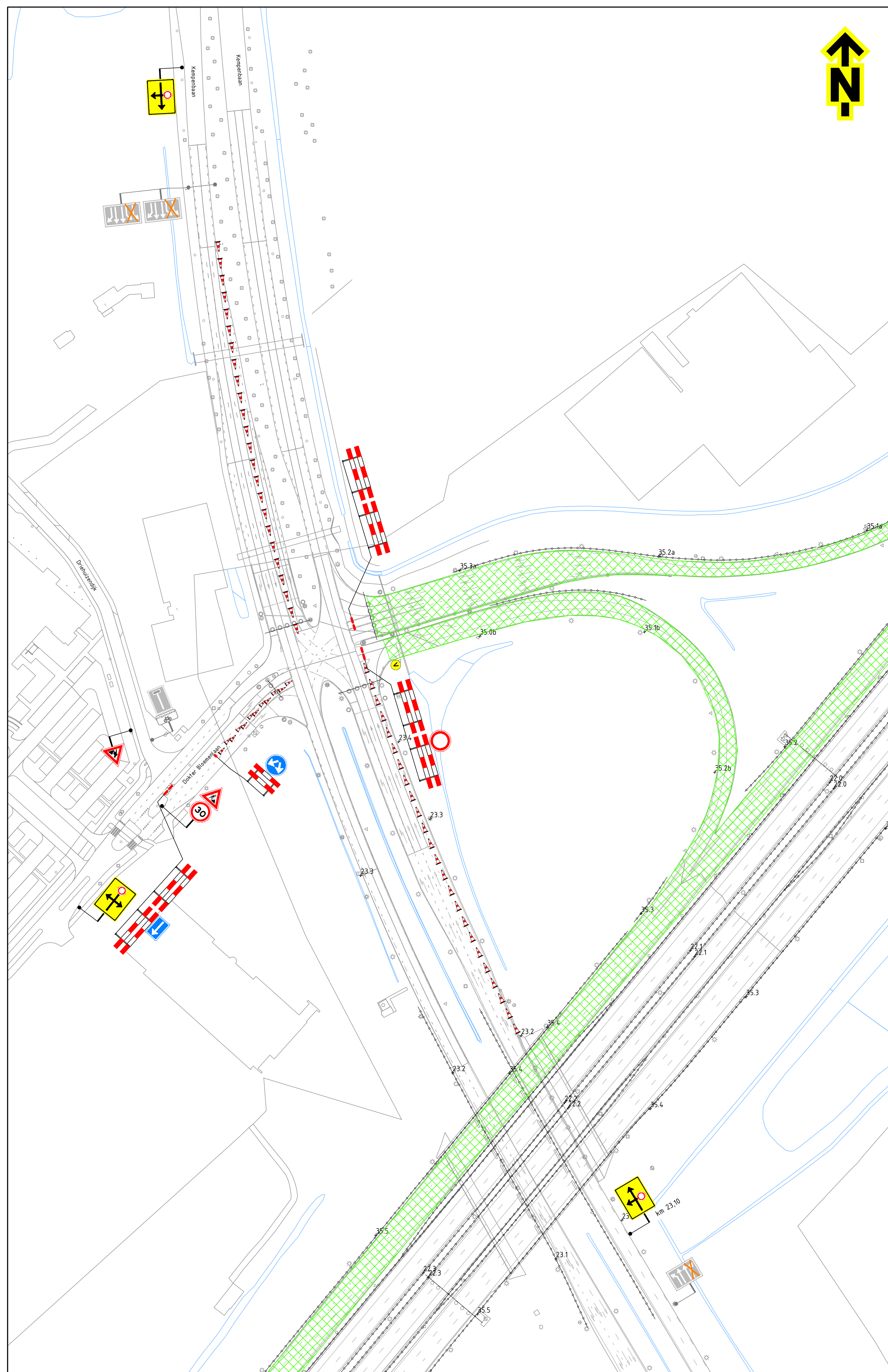
DETAIL SCHAAL 1 : 1.000 1 -
