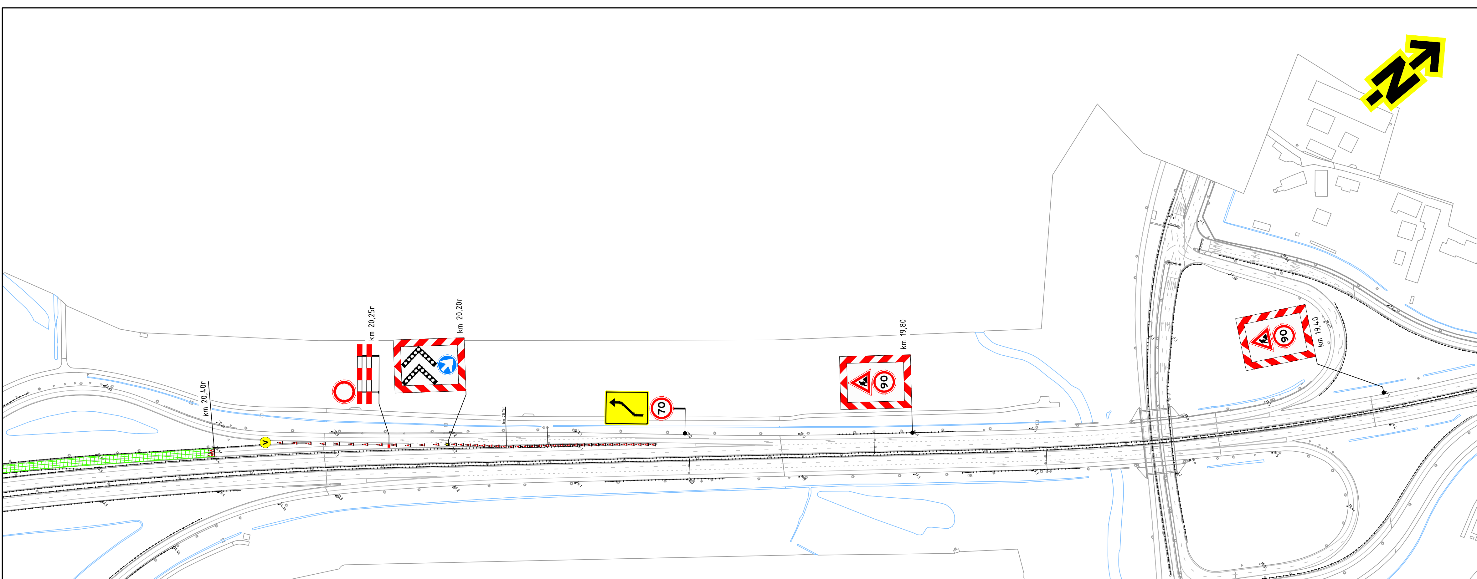
DETAIL 2 SCHAAL 1 : 2.000
