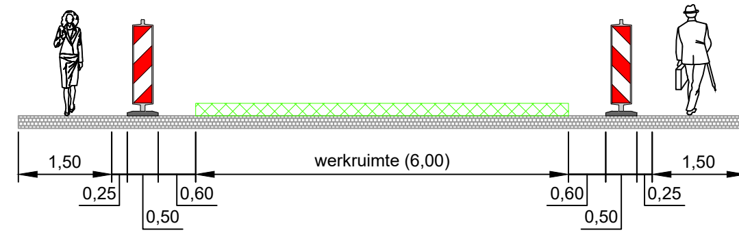
Dwarsprofiel A
