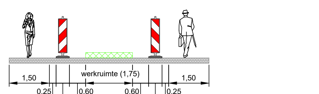
Dwarsprofiel C
