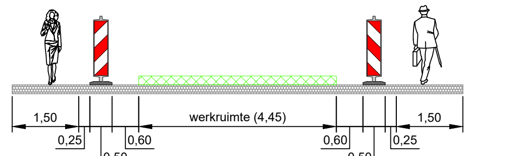
Dwarsprofiel B
