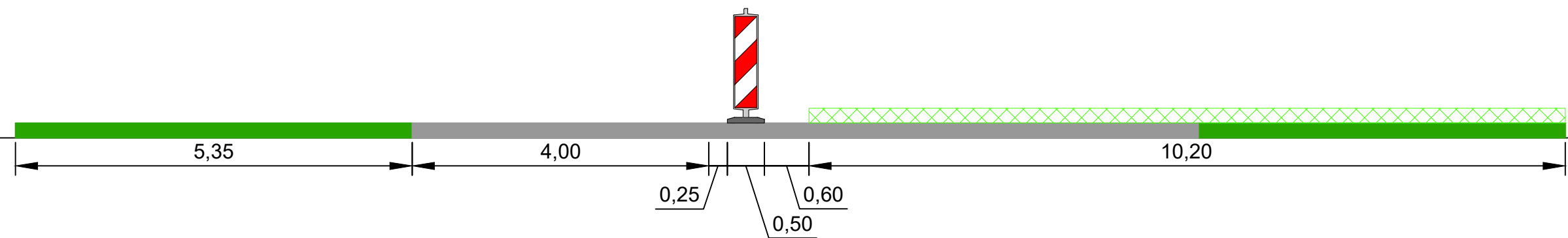
Dwarsprofiel A-A
