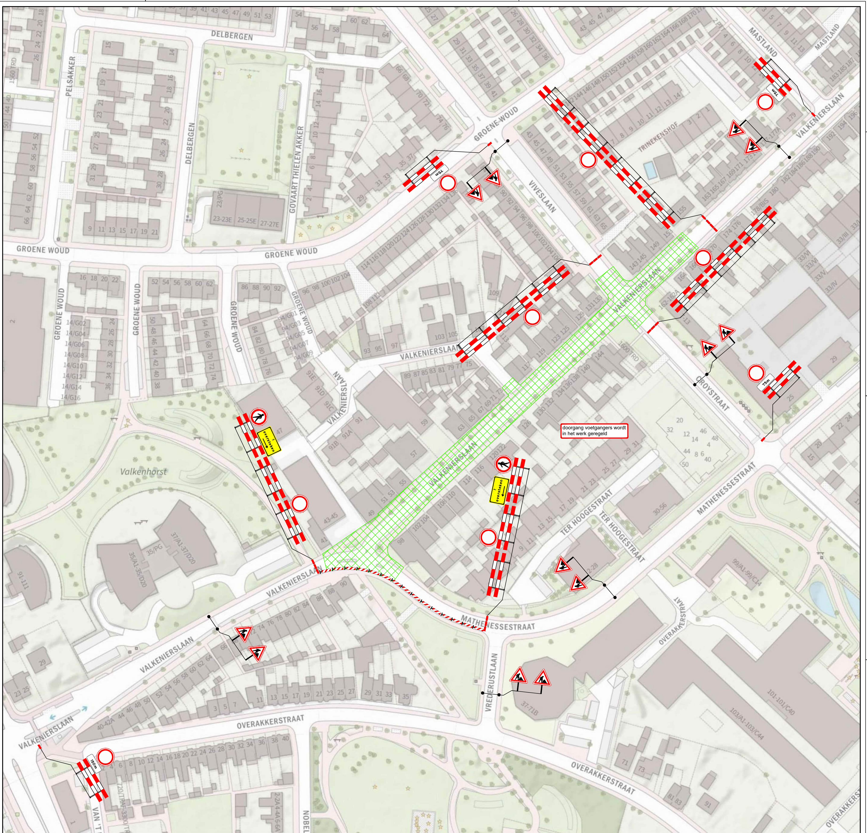
DETAIL 1 afzettingstekening
