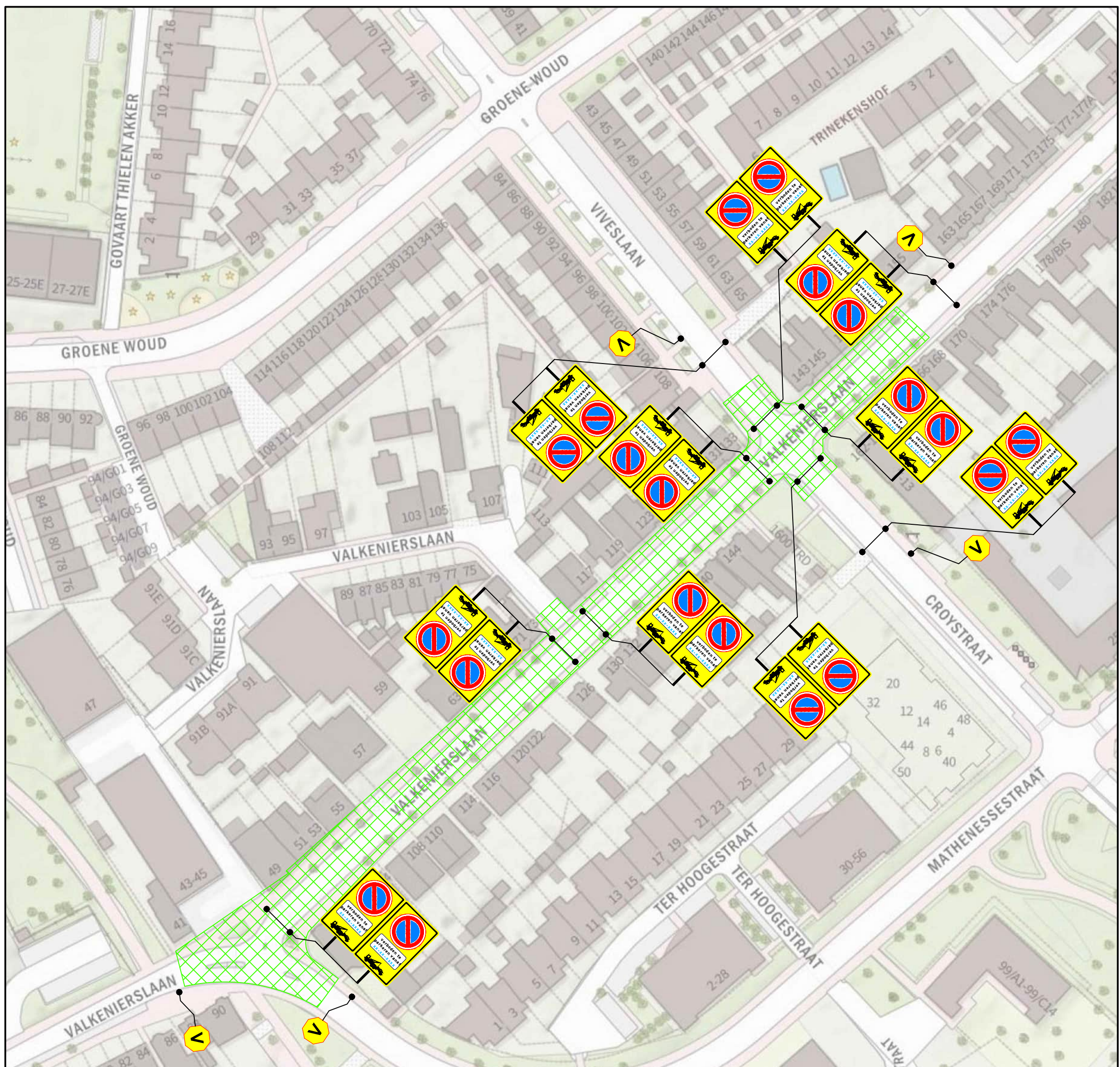
DETAIL 2 parkeerverboden & VA
