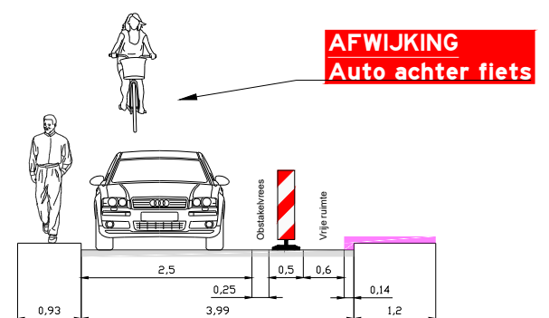
Dwarsprofiel B Schaal: 1:100
