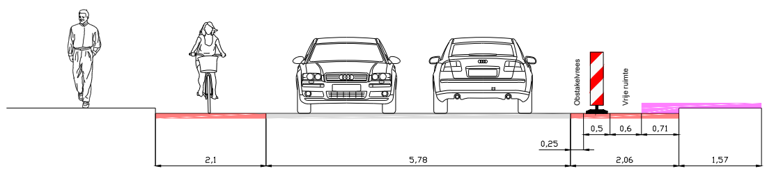
Dwarsprofiel B Schaal: 1:100
